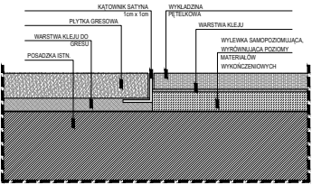
SZCZEGÓŁ LICOWANIA MATERIAŁÓW WYKOŃCZENIOWYCH POSADZKI W PRZYPADKU ICH RÓŻNEJ GRUBOŚCI
