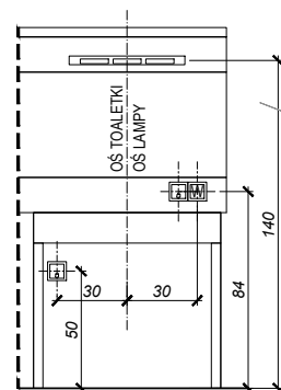
SCHEMAT ROZMIESZCZENIA ZESTAWU ELEKTRYCZNEGO DLA POJEDYNCZEGO STANOWISKA TOALETKI Z LUSTREM
