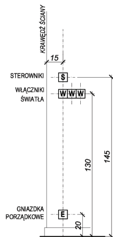
SCHEMAT ROZMIESZCZENIA URZĄDZEŃ ELEKTRYCZNYCH
