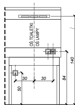
SCHEMAT ROZMIESZCZENIA ZESTAWU ELEKTRYCZNEGO DLA POJEDYŃCZEGO STANOWISKA TOALETKI Z LUSTREM
